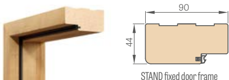
STAND fixed door frame
