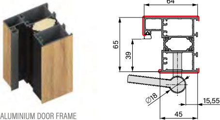
ALUMINIUM DOOR FRAME
