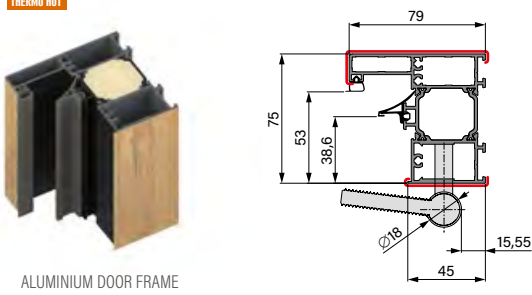
ALUMINIUM DOOR FRAME
