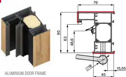
ALUMINIUM DOOR FRAME
