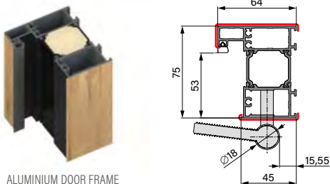
ALUMINIUM DOOR FRAME
